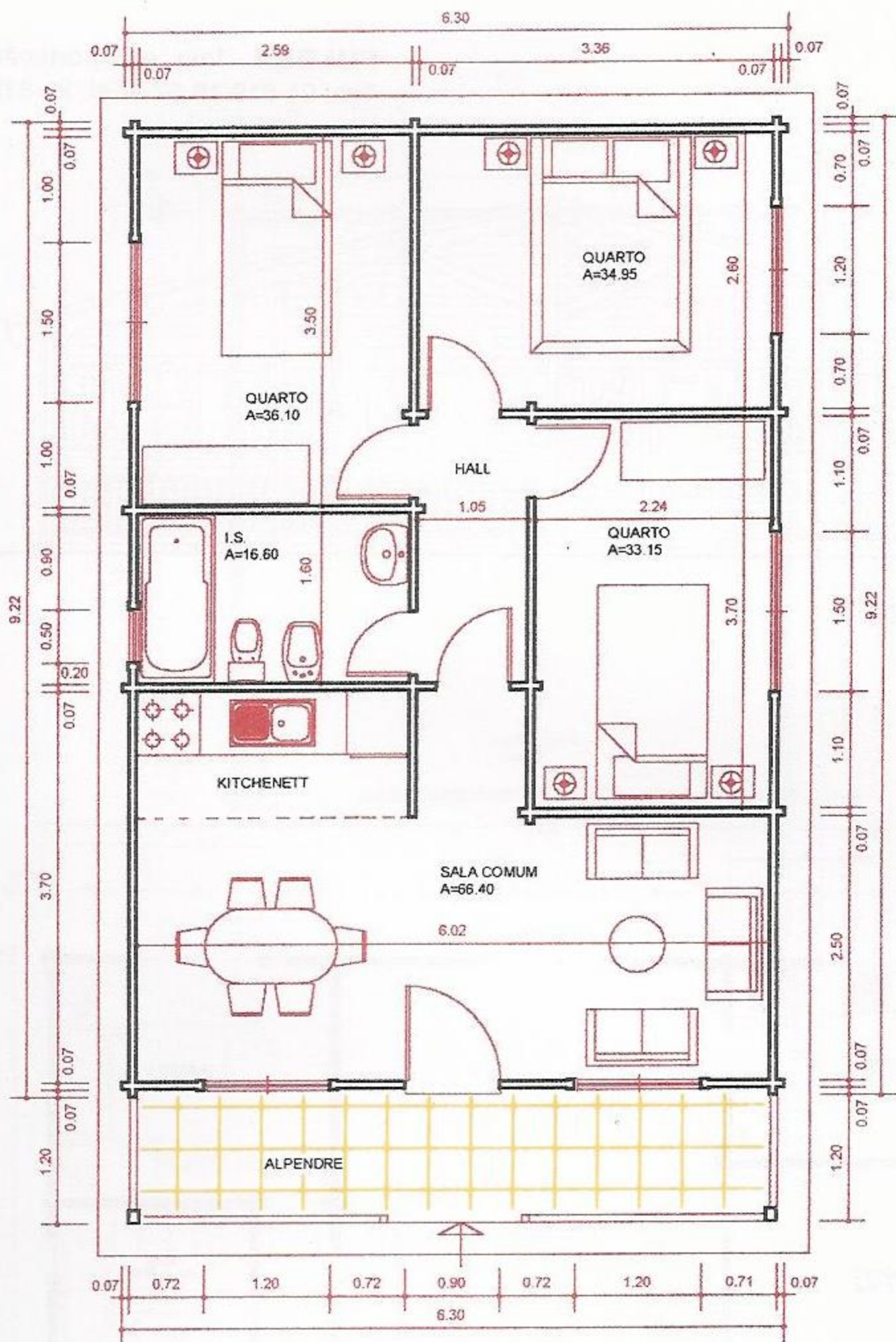
PLANTA
