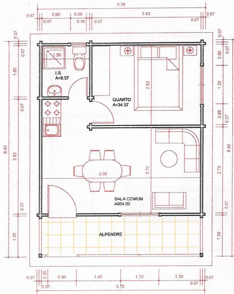
PLANTA
