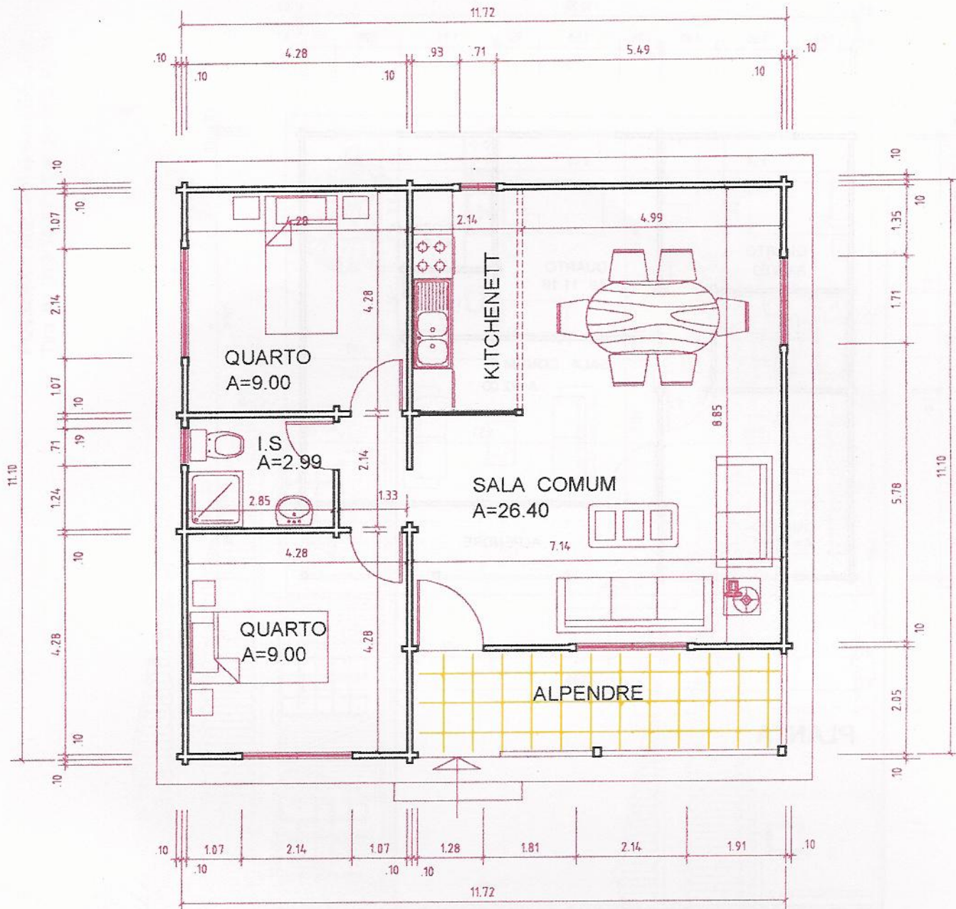
PLANTA
