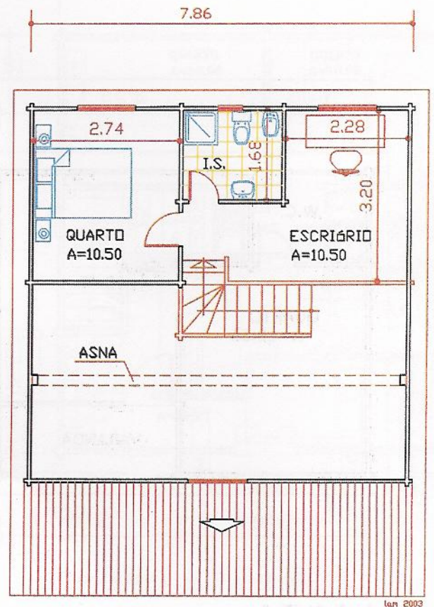
PLANTA do piso 1 ( A=28.79 m 2 )
